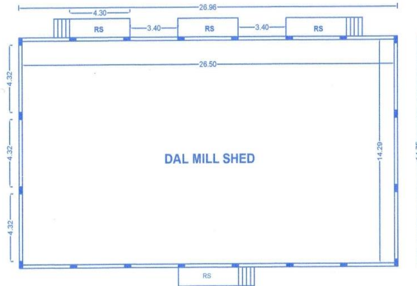
PLAN FOR DAL MILL SHED
